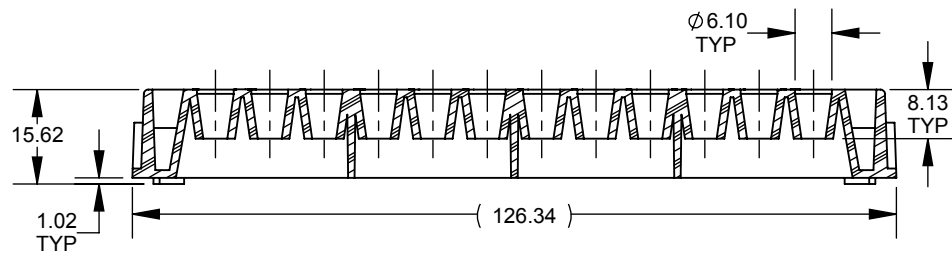
SECTION A-A SCALE: 0.8 : 1
