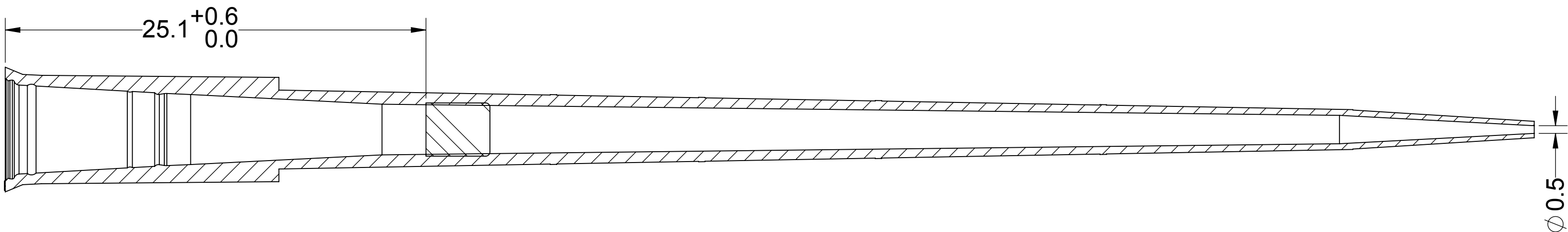
SECTION A-A
