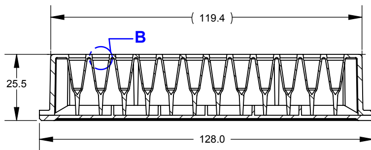
SECTION A-A SCALE: 0.7 : 1
