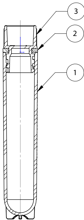
SECTION A-A
